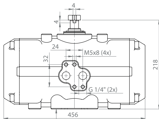
Ansicht / view A
